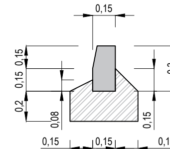
Kelio bordiūro su pamatu detalė 100x15x30
