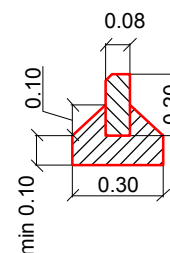
Detalė "A" Vejos bortas 100x20x8 M 1:20
