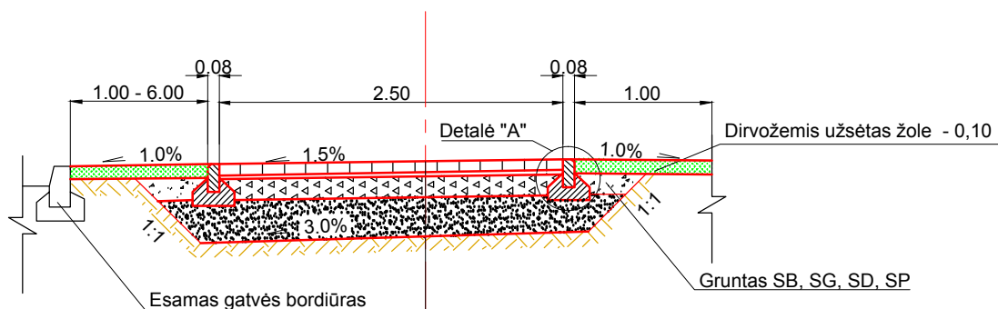
Tipas I I - II etapai Pk 0+00 - Pk 16+96
