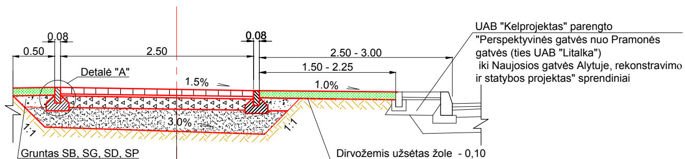
Tipas III III etapas Pk 2+13 - Pk 4+82.50
