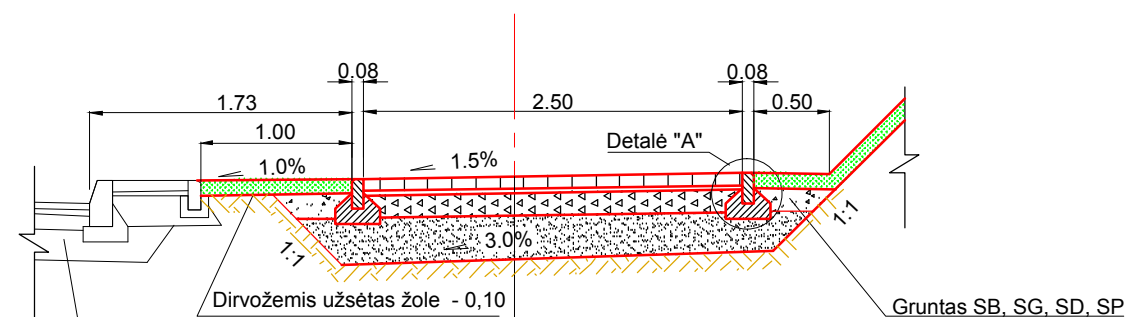
Tipas II III etapas Pk 0+00 - Pk 2+13
