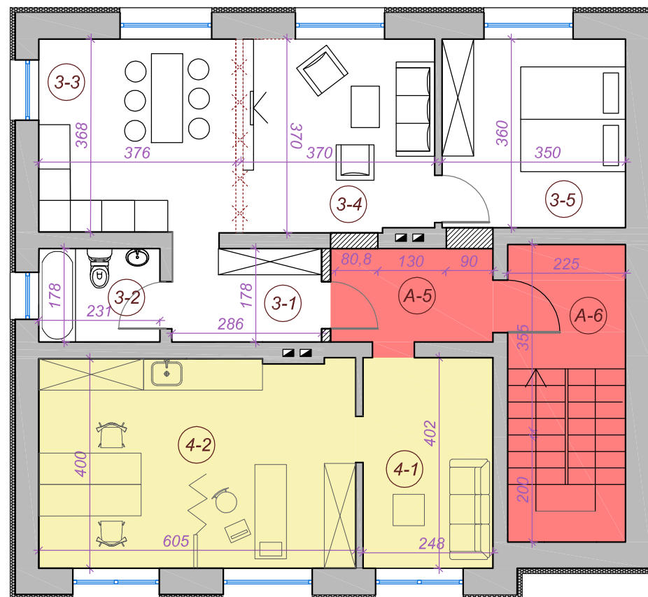
ANTRO AUKŠTO PLANAS M 1:100
