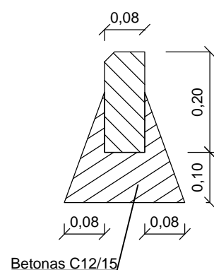
Betoninis vejos bordiūras M 1:10
