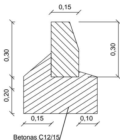
Betoninis kelio bordiūras M 1:10
